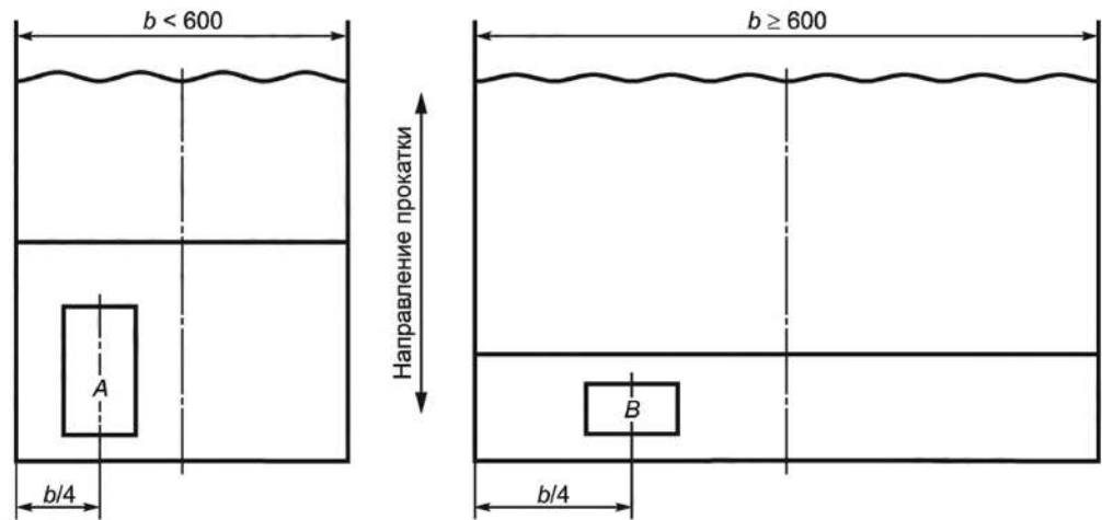
b — ширина проката; A и B — место отбора проб
